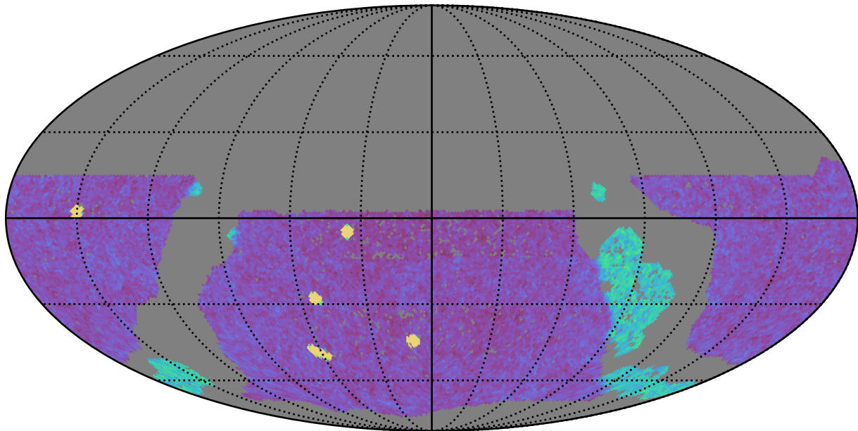
mw_roll_all_v3.3_10yrs WFD g band: NVisits
