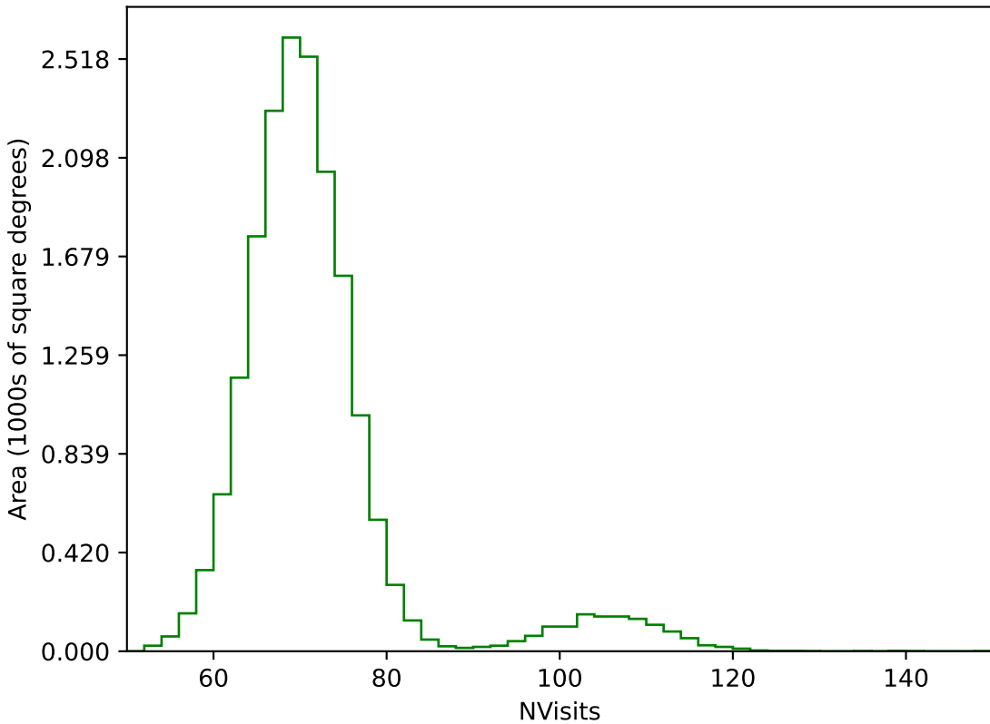
mw_roll_all_v3.3_10yrs WFD g band: NVisits
