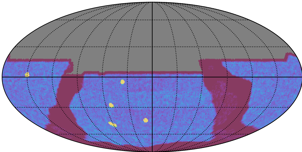
mw_roll_all_v3.3_10yrs All sky y band: NVisits
