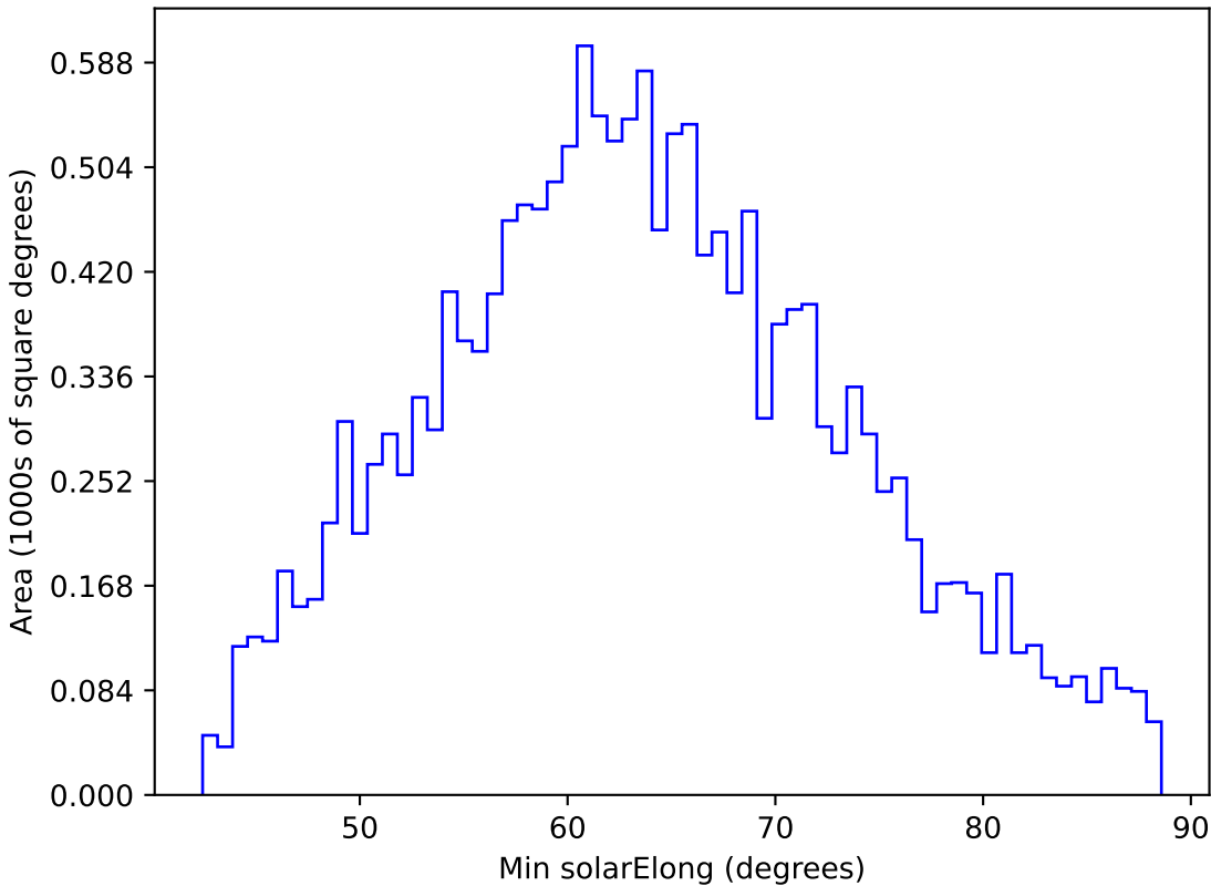
mw_roll_all_v3.3_10yrs WFD y band: Min solarElong
