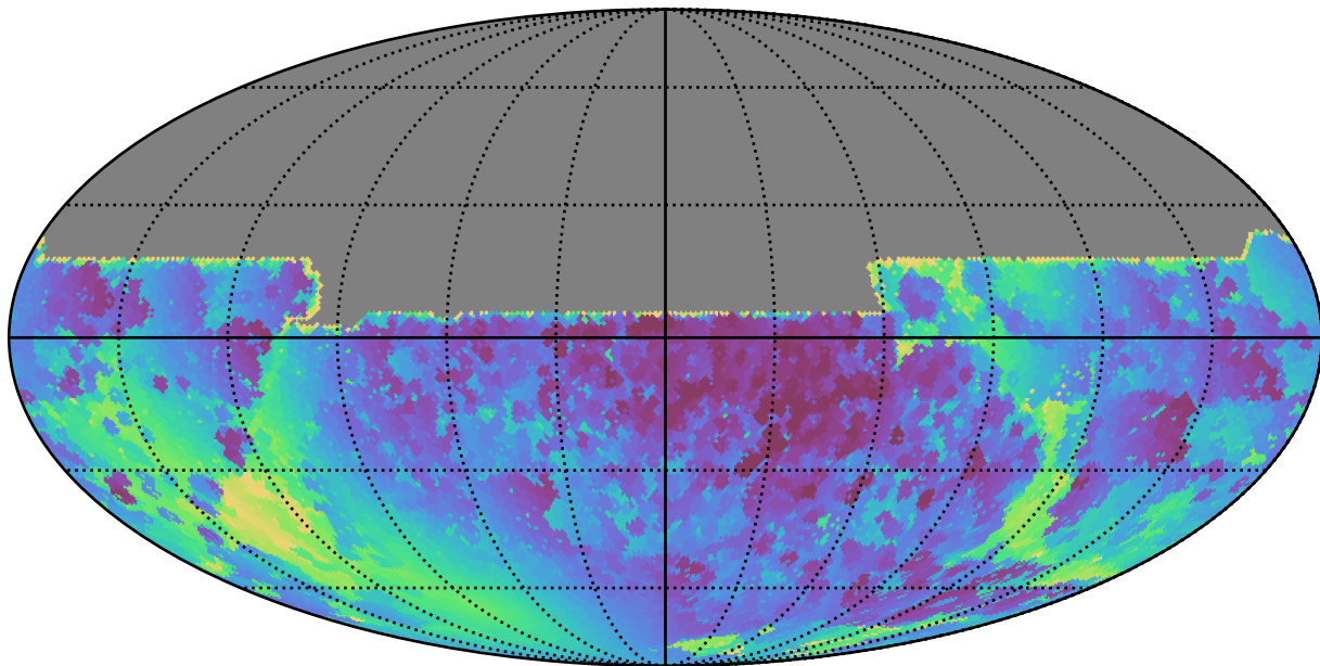
mw_roll_all_v3.3_10yrs All sky y band: Min solarElong
