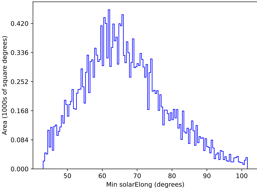
mw_roll_all_v3.3_10yrs All sky y band: Min solarElong
