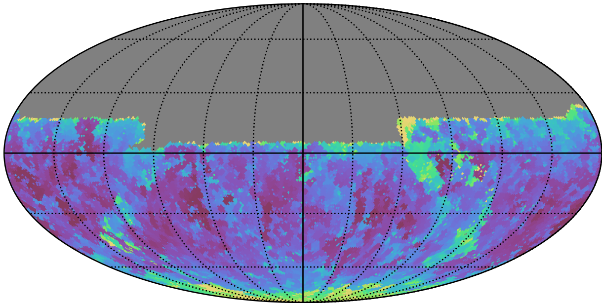
mw_roll_all_v3.3_10yrs Yr 1 y band: Min seeingGeom
