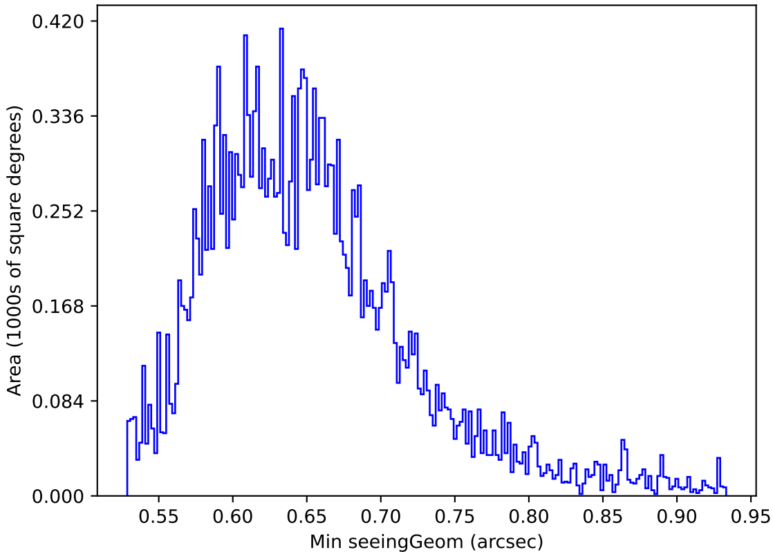
mw_roll_all_v3.3_10yrs Yr 1 y band: Min seeingGeom
