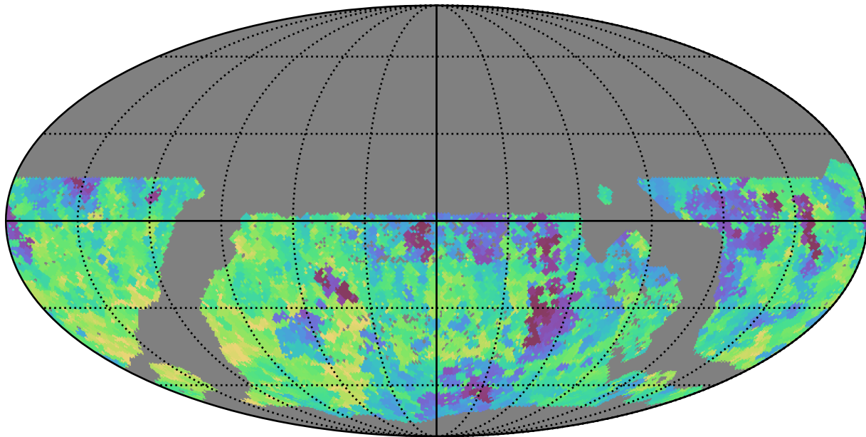
mw_roll_all_v3.3_10yrs WFD z band: Min saturation_mag
