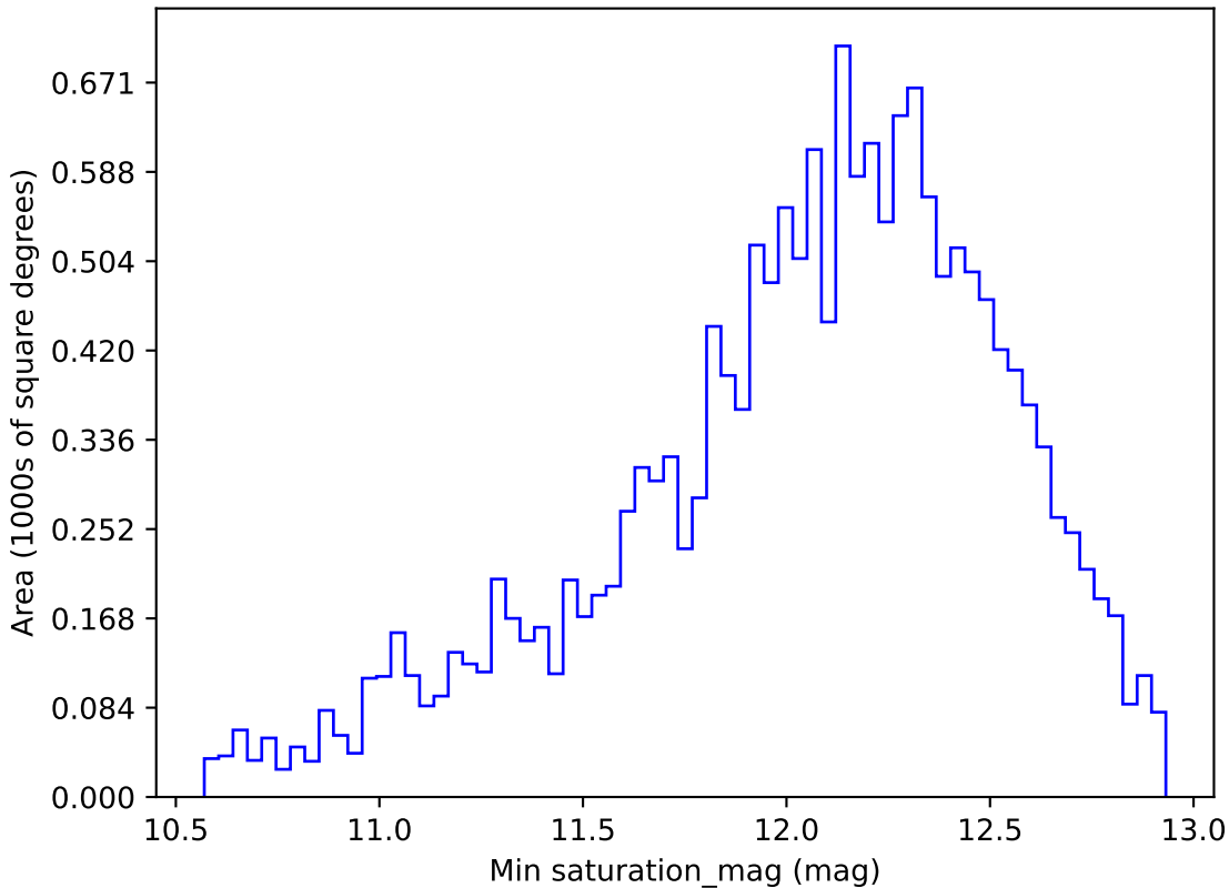
mw_roll_all_v3.3_10yrs WFD z band: Min saturation_mag
