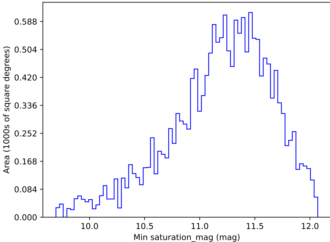
mw_roll_all_v3.3_10yrs WFD y band: Min saturation_mag
