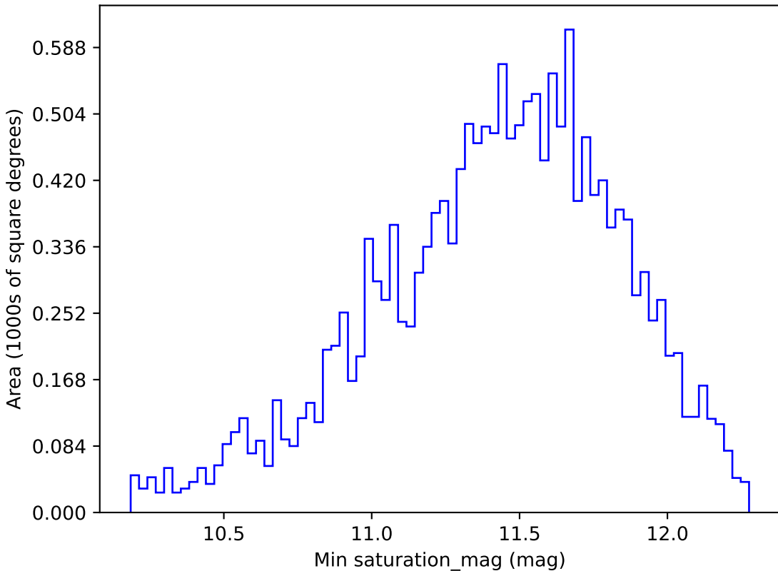
mw_roll_all_v3.3_10yrs WFD u band: Min saturation_mag
