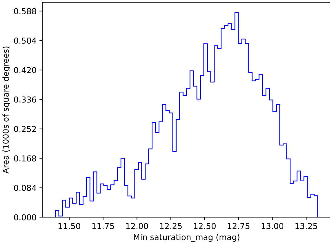
mw_roll_all_v3.3_10yrs WFD r band: Min saturation_mag
