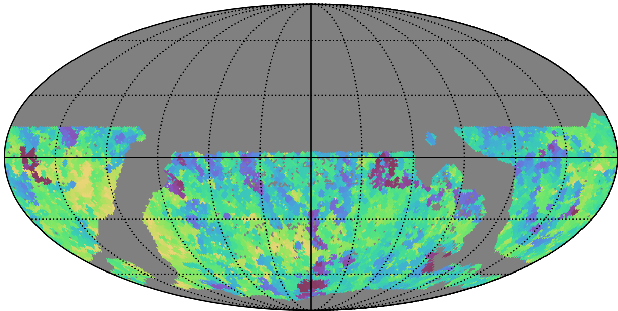
mw_roll_all_v3.3_10yrs WFD i band: Min saturation_mag
