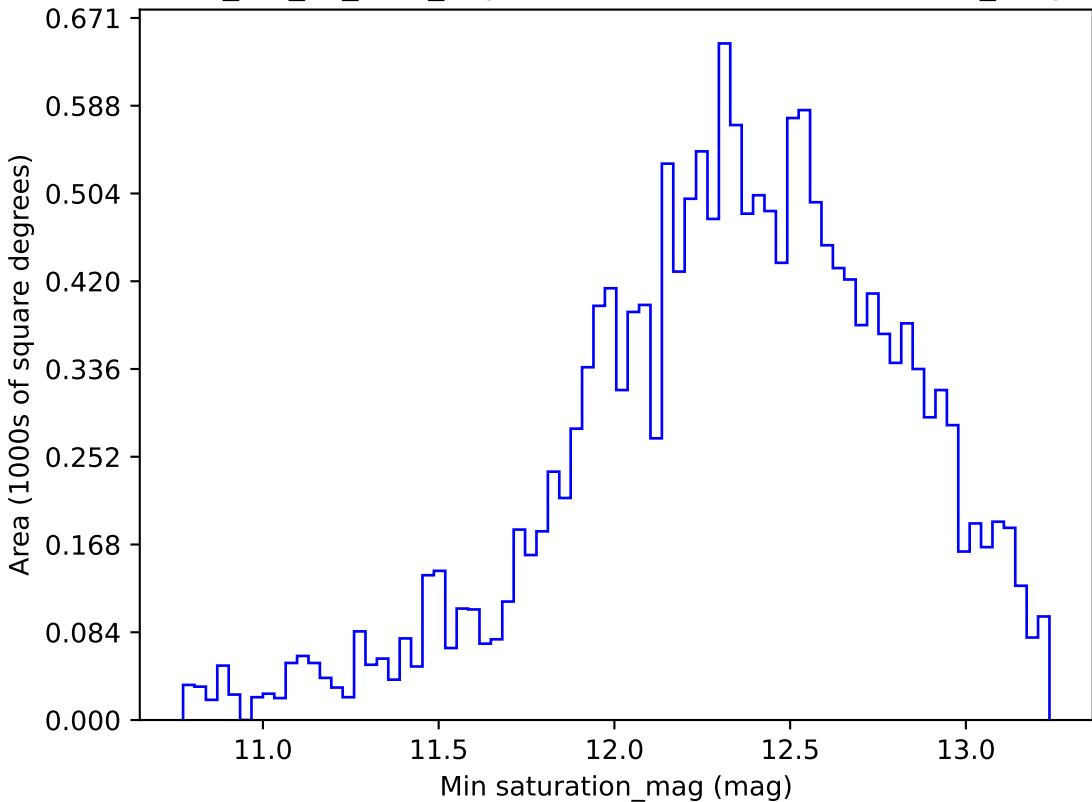
mw_roll_all_v3.3_10yrs WFD i band: Min saturation_mag
