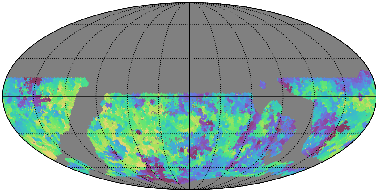
mw_roll_all_v3.3_10yrs WFD g band: Min saturation_mag
