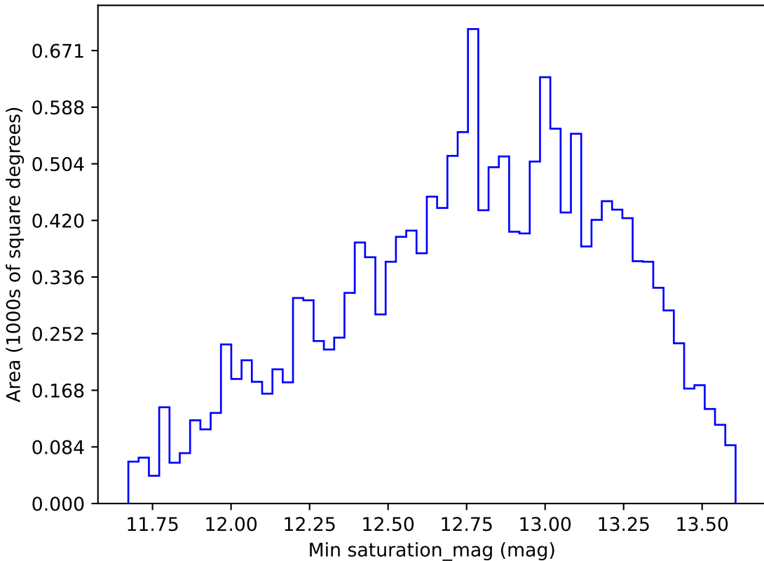
mw_roll_all_v3.3_10yrs WFD g band: Min saturation_mag
