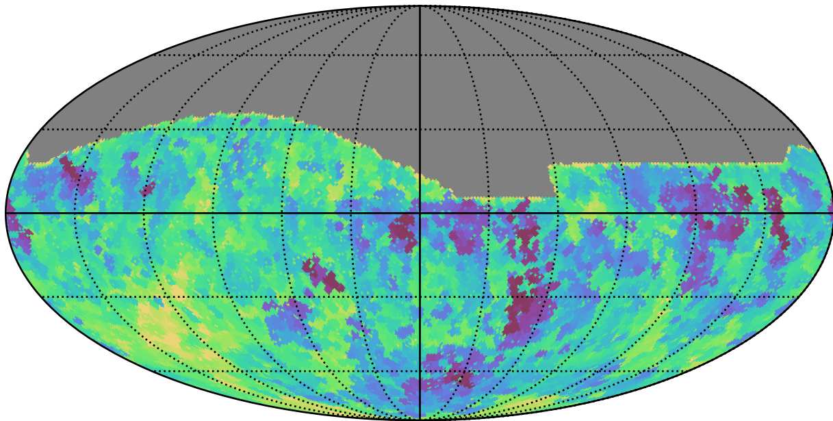
mw_roll_all_v3.3_10yrs All sky z band: Min saturation_mag
