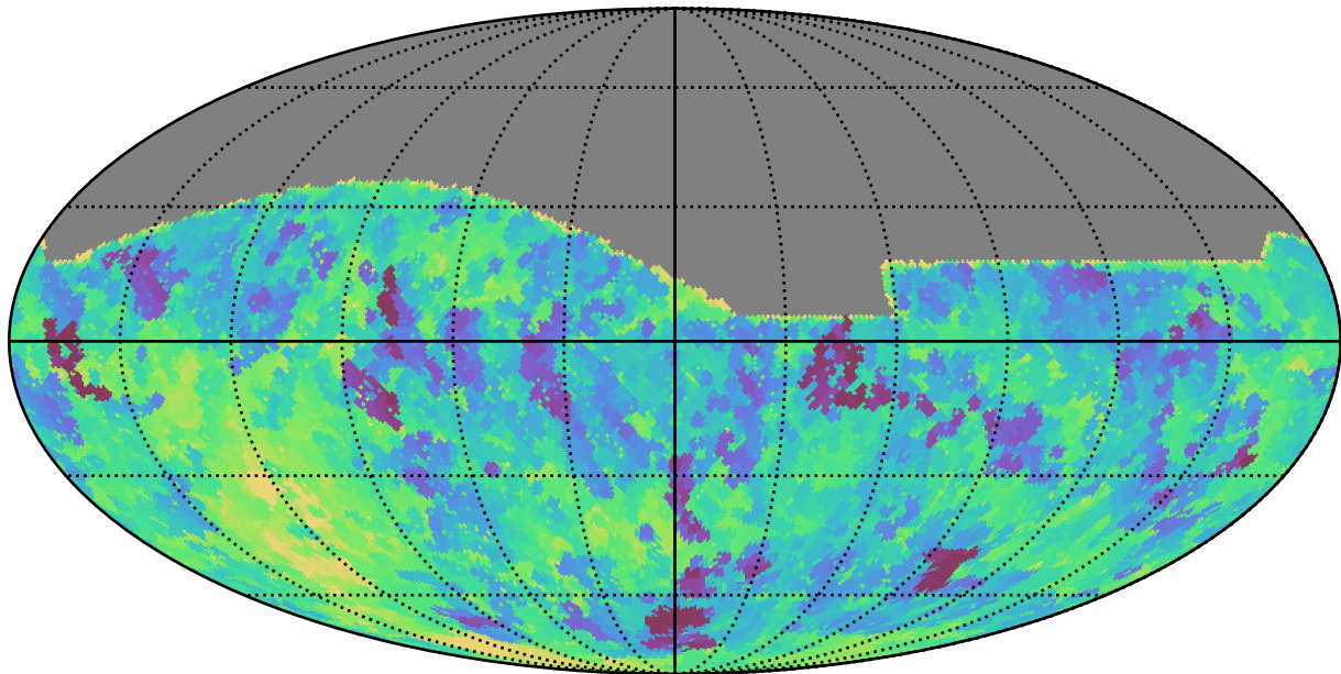
mw_roll_all_v3.3_10yrs All sky i band: Min saturation_mag
