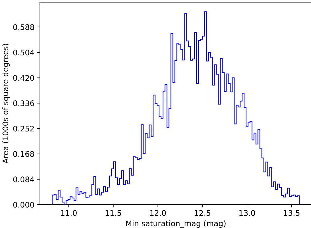
mw_roll_all_v3.3_10yrs All sky i band: Min saturation_mag
