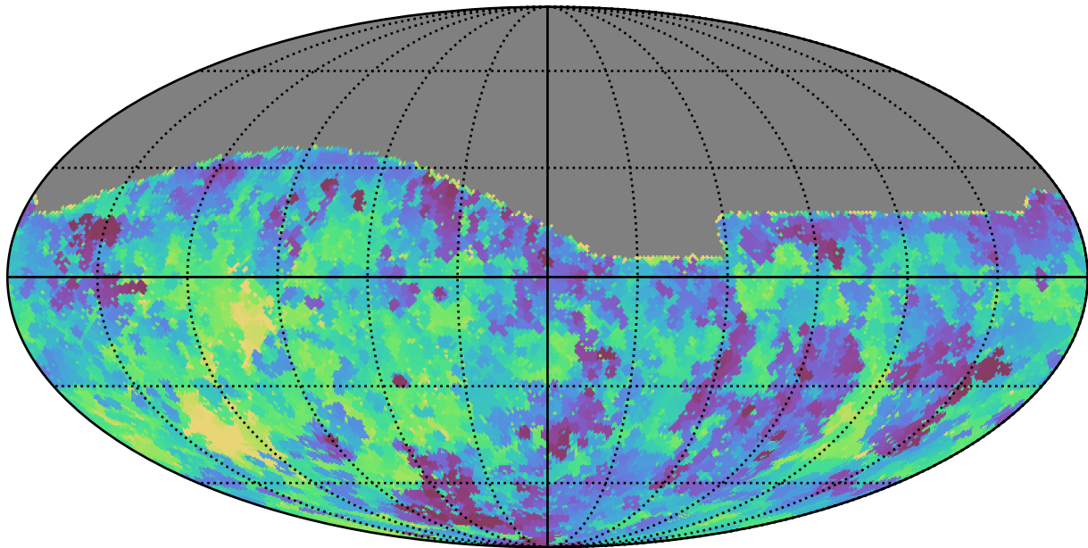
mw_roll_all_v3.3_10yrs All sky g band: Min saturation_mag
