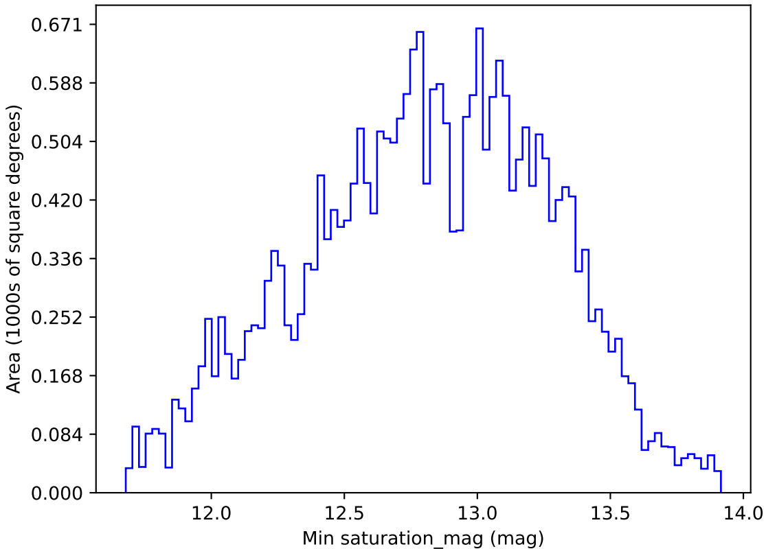
mw_roll_all_v3.3_10yrs All sky g band: Min saturation_mag
