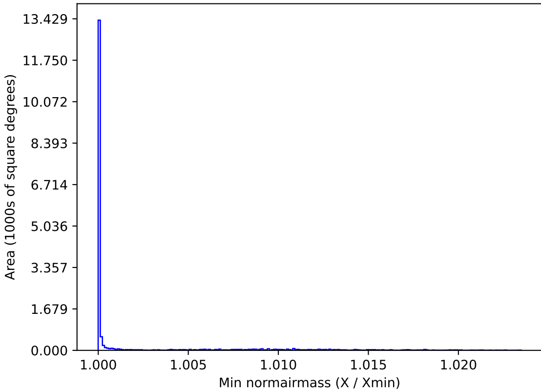
mw_roll_all_v3.3_10yrs WFD z band: Min normairmass
