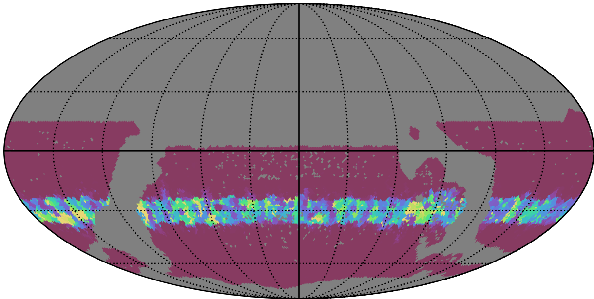
mw_roll_all_v3.3_10yrs WFD y band: Min normairmass
