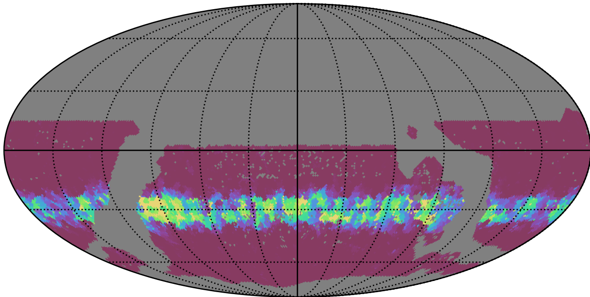
mw_roll_all_v3.3_10yrs WFD u band: Min normairmass
