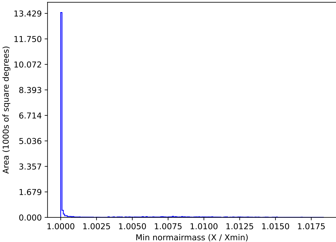
mw_roll_all_v3.3_10yrs WFD r band: Min normairmass
