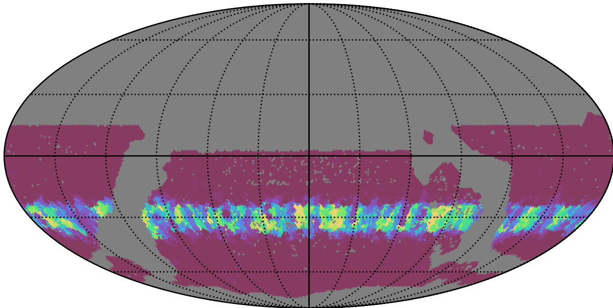
mw_roll_all_v3.3_10yrs WFD g band: Min normairmass
