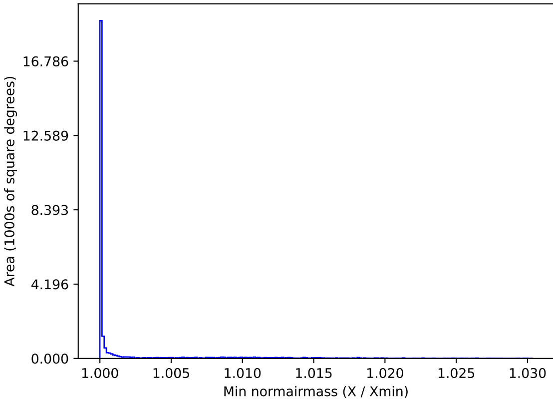
mw_roll_all_v3.3_10yrs All sky z band: Min normairmass
