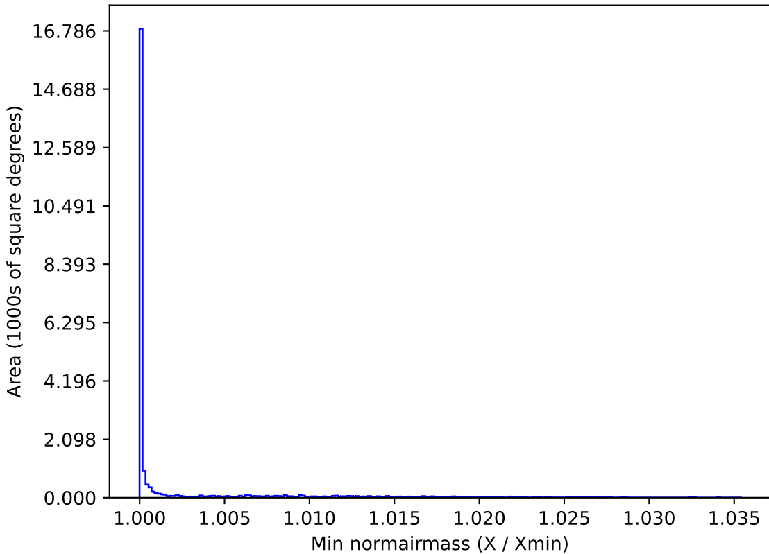
mw_roll_all_v3.3_10yrs All sky y band: Min normairmass
