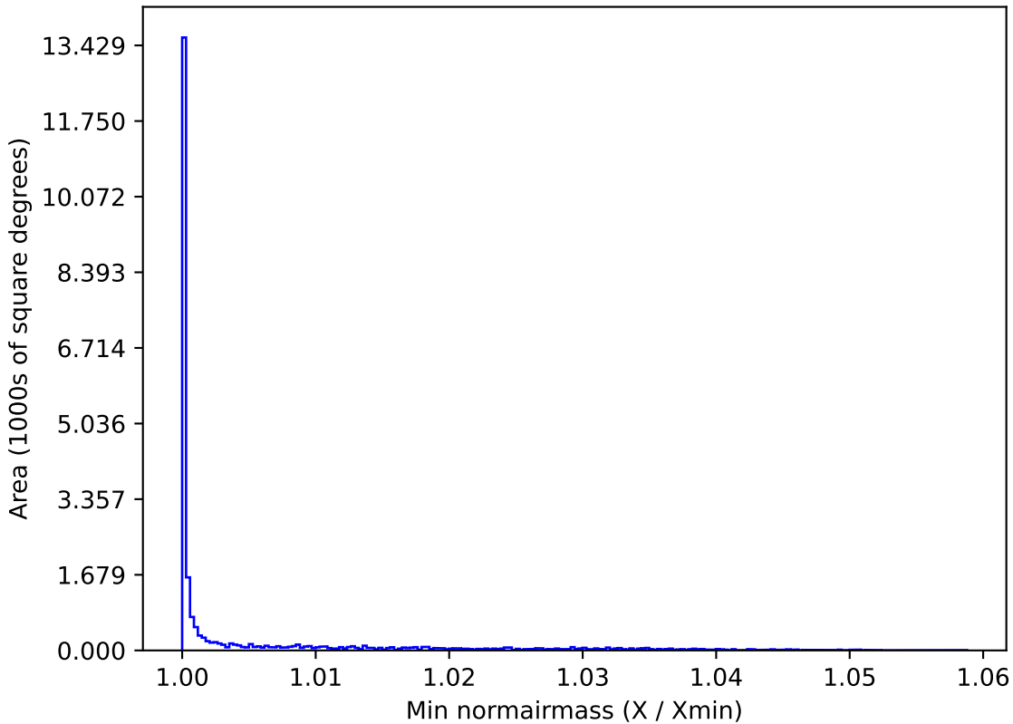
mw_roll_all_v3.3_10yrs All sky u band: Min normairmass
