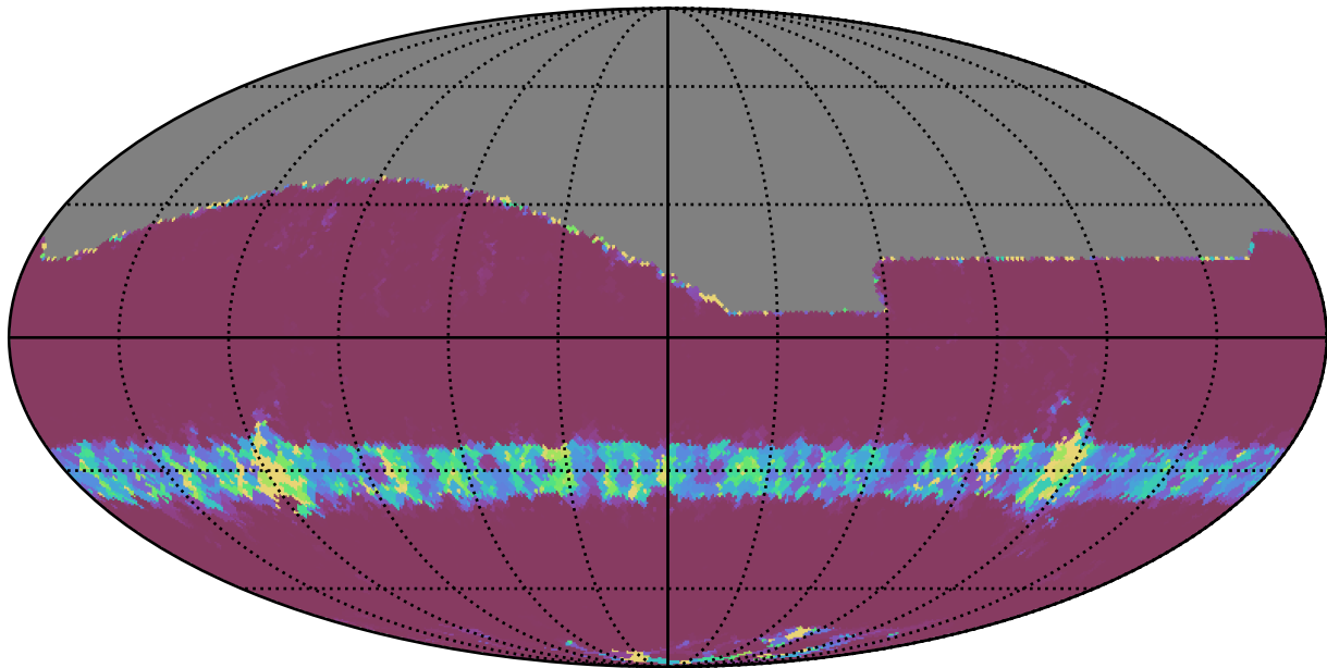
mw_roll_all_v3.3_10yrs All sky r band: Min normairmass
