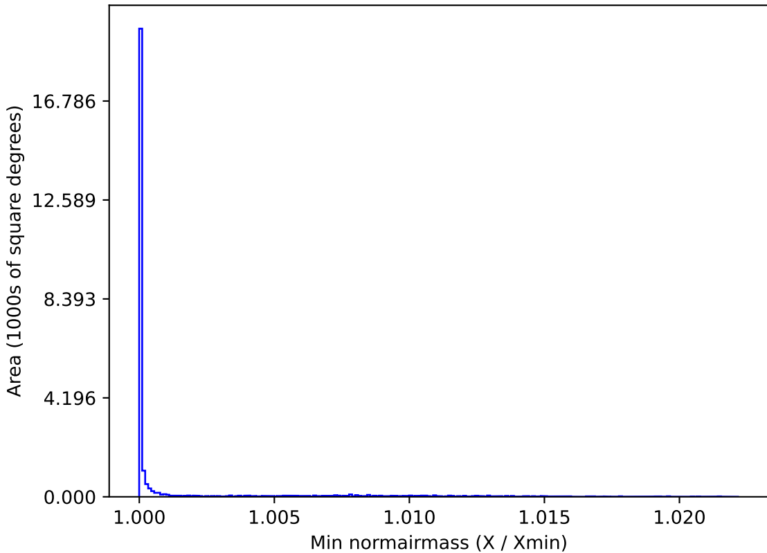
mw_roll_all_v3.3_10yrs All sky r band: Min normairmass
