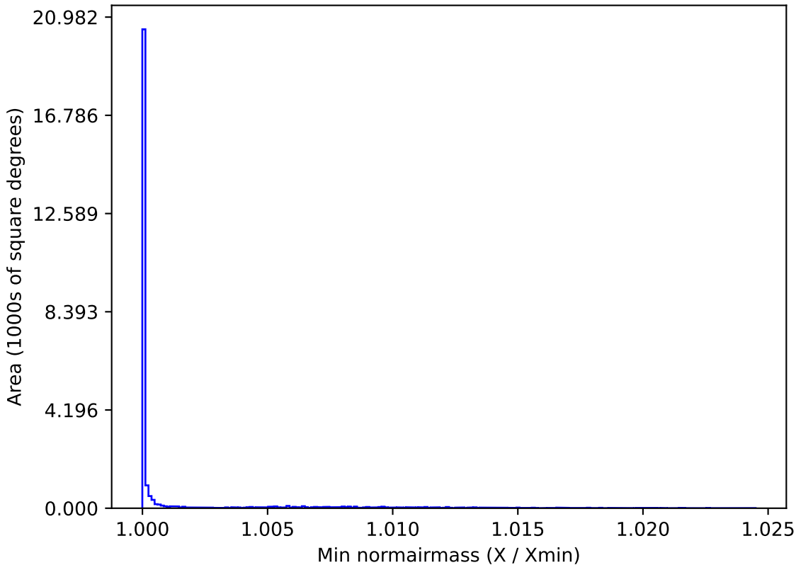
mw_roll_all_v3.3_10yrs All sky i band: Min normairmass
