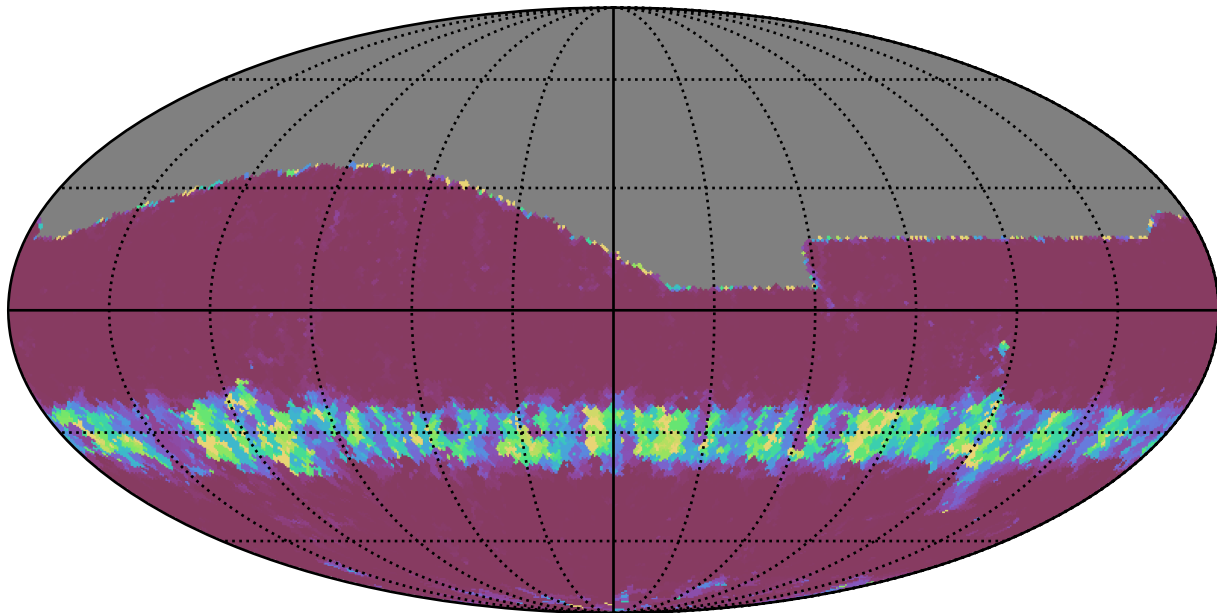
mw_roll_all_v3.3_10yrs All sky g band: Min normairmass
