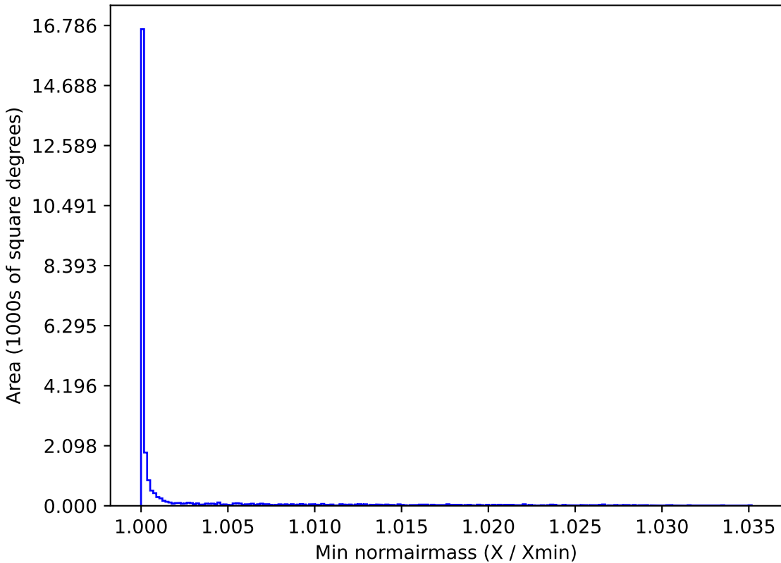
mw_roll_all_v3.3_10yrs All sky g band: Min normairmass
