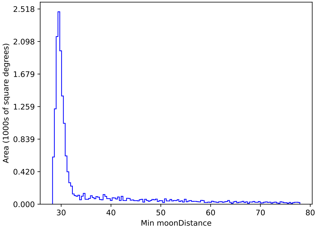
mw_roll_all_v3.3_10yrs WFD z band: Min moonDistance
