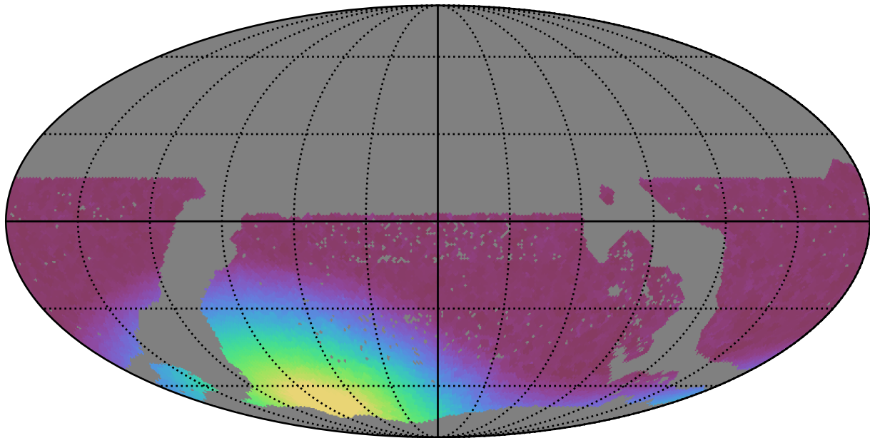
mw_roll_all_v3.3_10yrs WFD y band: Min moonDistance
