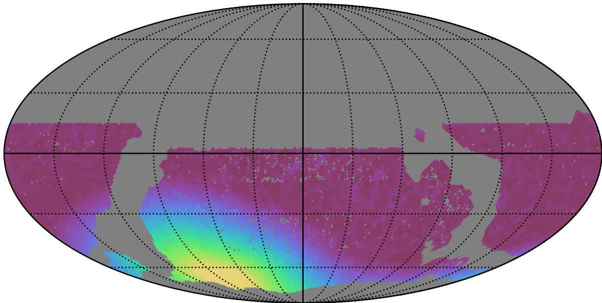
mw_roll_all_v3.3_10yrs WFD i band: Min moonDistance
