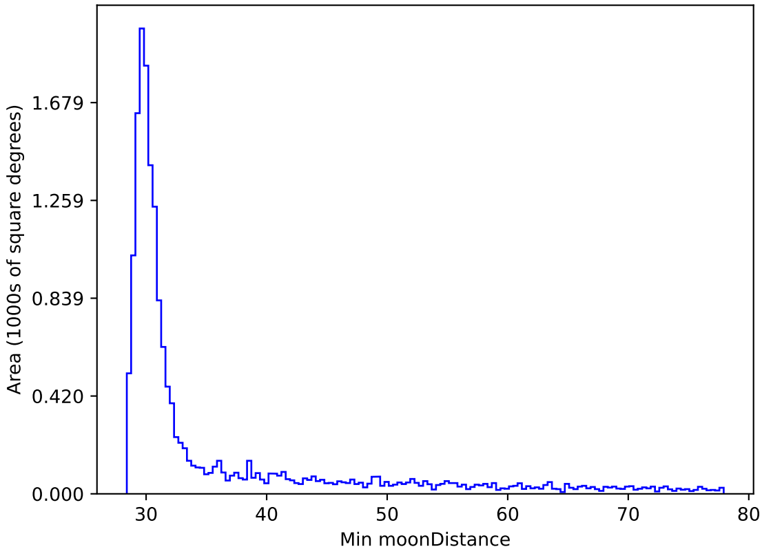
mw_roll_all_v3.3_10yrs WFD i band: Min moonDistance
