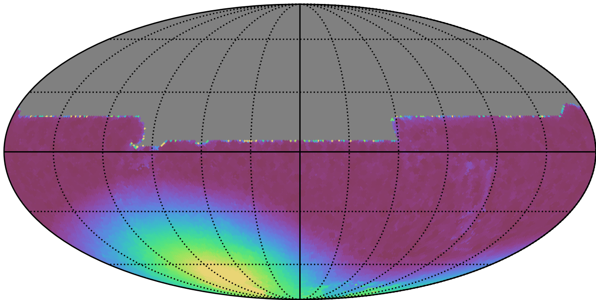
mw_roll_all_v3.3_10yrs All sky y band: Min moonDistance
