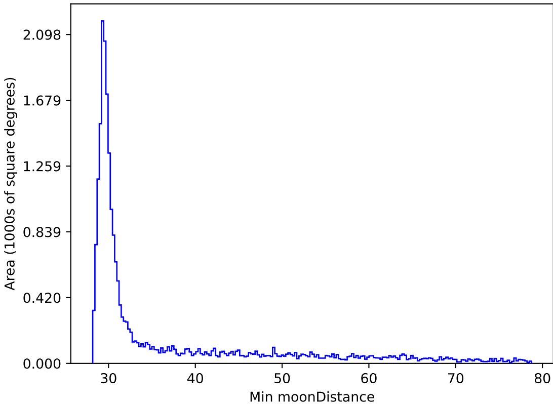
mw_roll_all_v3.3_10yrs All sky y band: Min moonDistance
