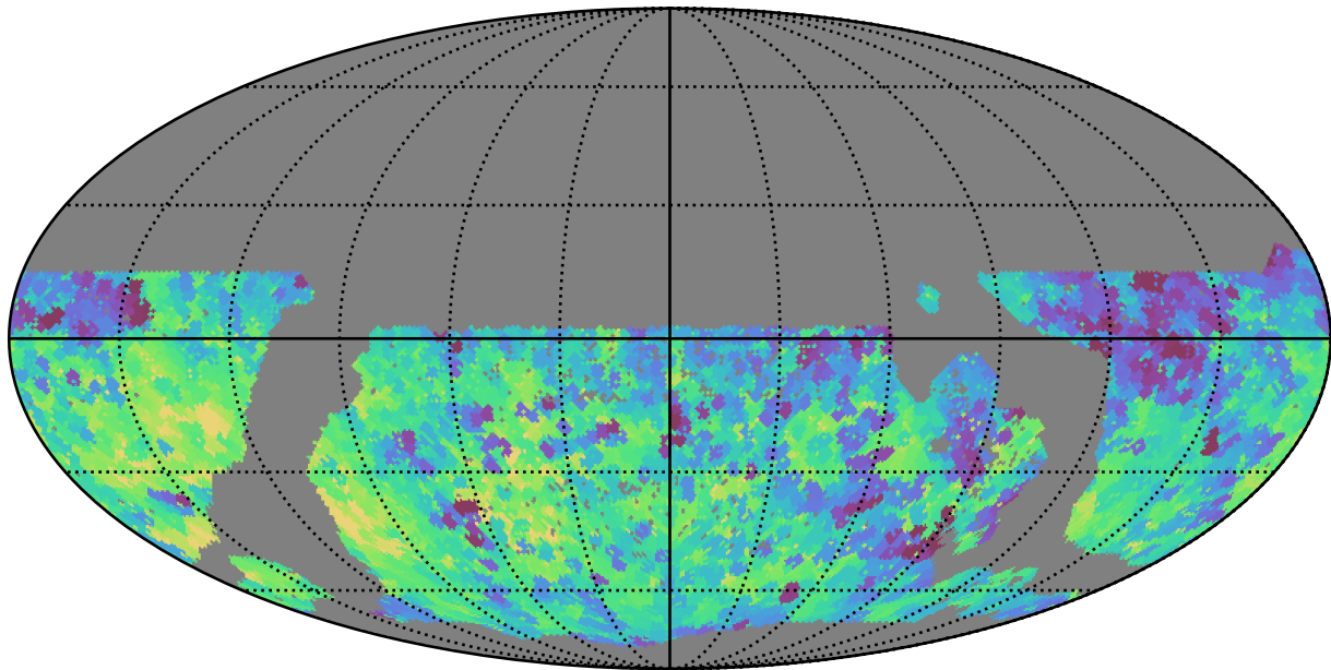
mw_roll_all_v3.3_10yrs WFD y band: Min fiveSigmaDepth
