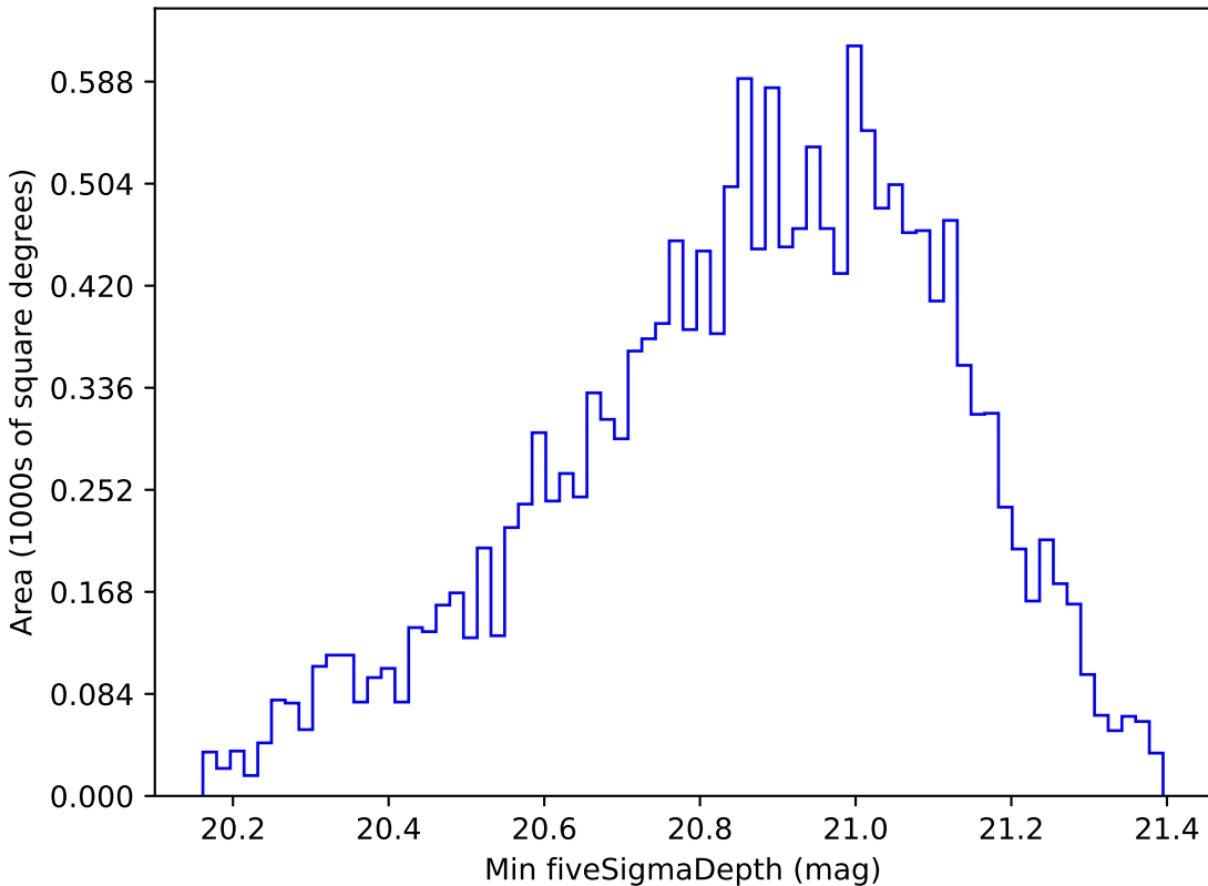
mw_roll_all_v3.3_10yrs WFD y band: Min fiveSigmaDepth
