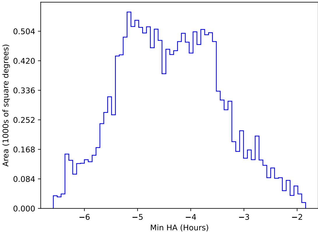
mw_roll_all_v3.3_10yrs WFD z band: Min HA
