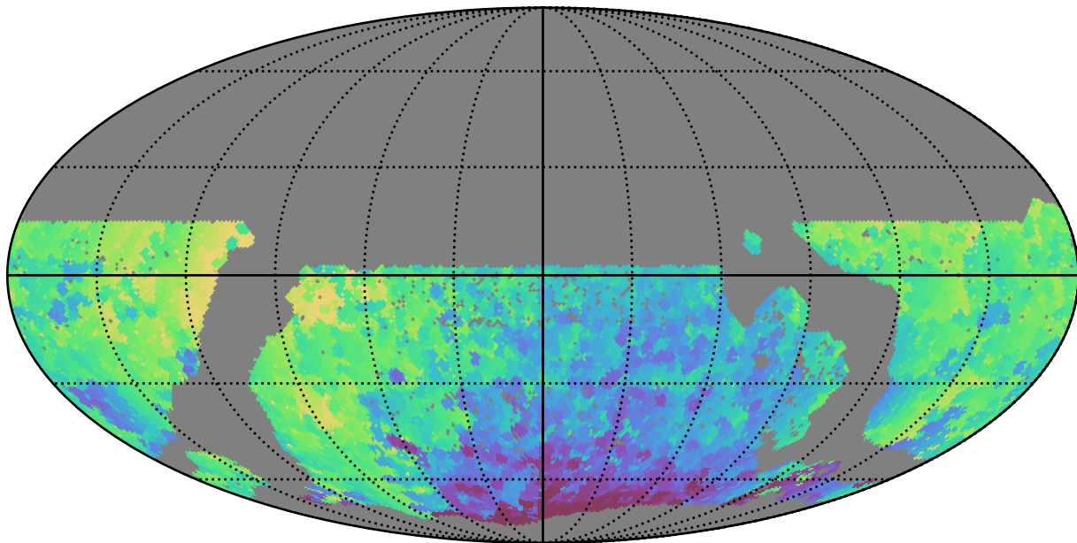
mw_roll_all_v3.3_10yrs WFD y band: Min HA
