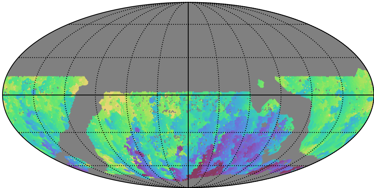
mw_roll_all_v3.3_10yrs WFD u band: Min HA
