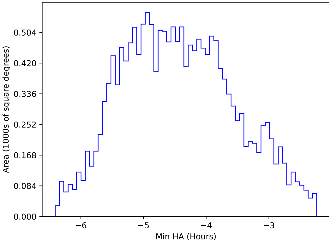
mw_roll_all_v3.3_10yrs WFD r band: Min HA
