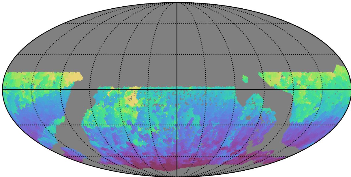
mw_roll_all_v3.3_10yrs WFD i band: Min HA
