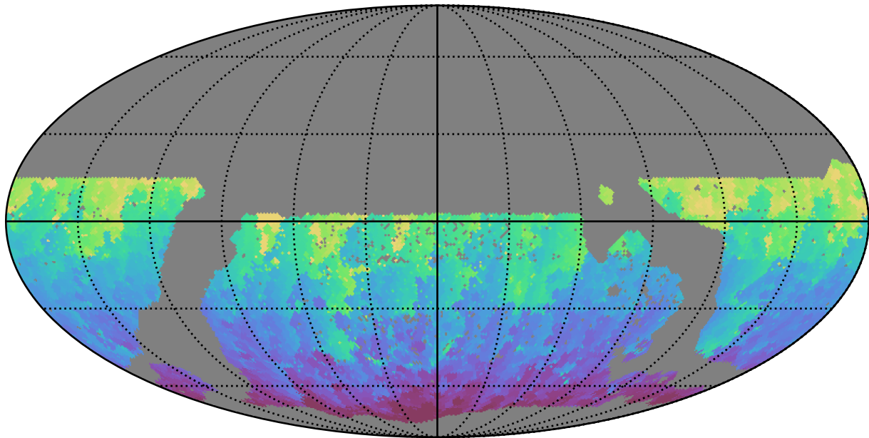
mw_roll_all_v3.3_10yrs WFD g band: Min HA
