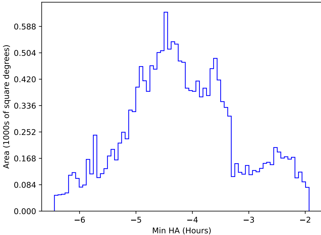
mw_roll_all_v3.3_10yrs WFD g band: Min HA
